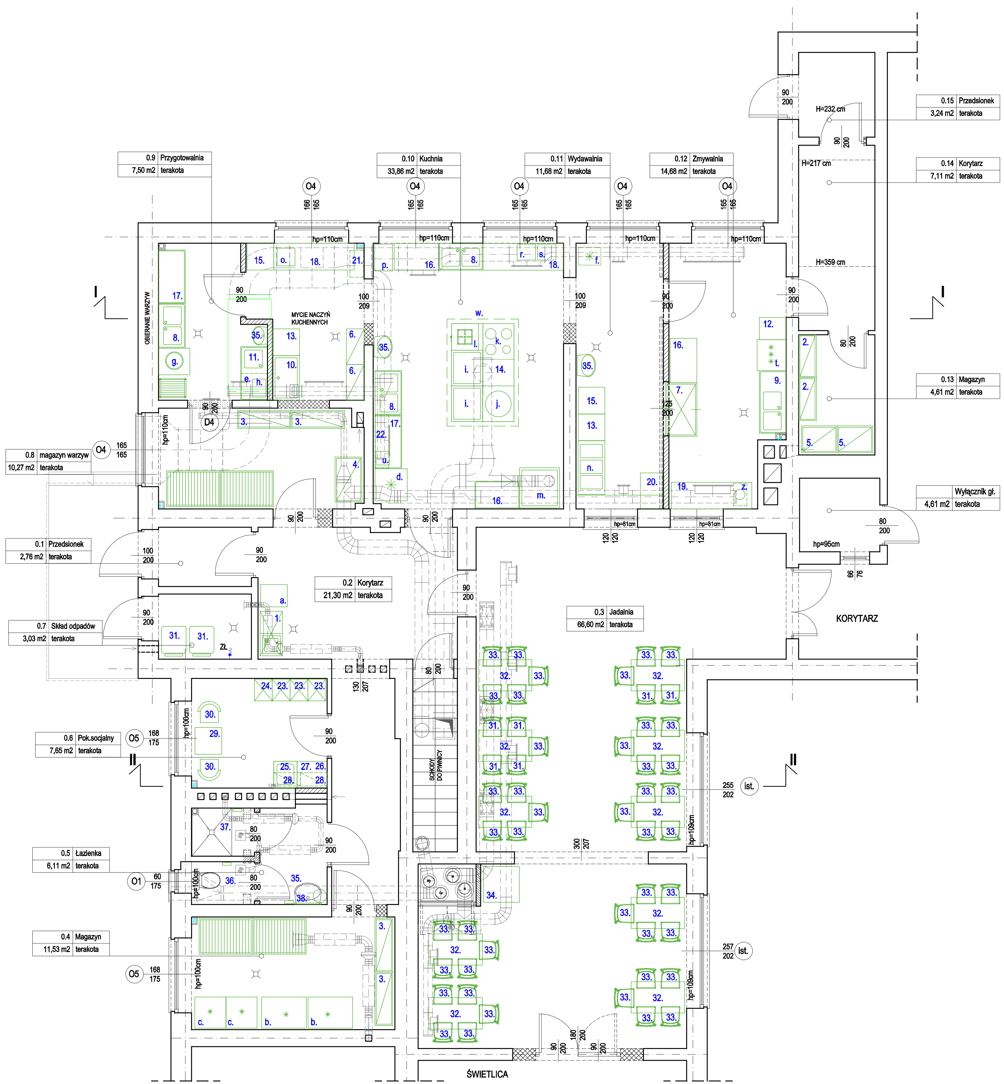
TECHNOLOGIA KUCHNI 1:50 RZUT PARTERU - ( fragment )
